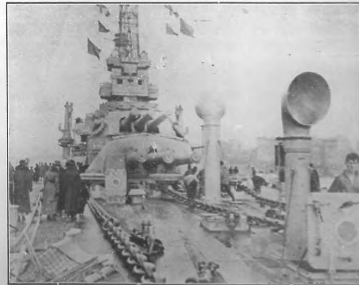
Vista del puente del acorazado "Pennsylvanía" mostrando los sus poderosos cañones de una de sus torres que obligaron a mantenerse embotellada a la escuadra alemana. Los americanos crean nuevas armas como las de los mares para vencer y aumentar infinitamente su comercio, no obstante ser partidarios de la Liga de Naciones.
